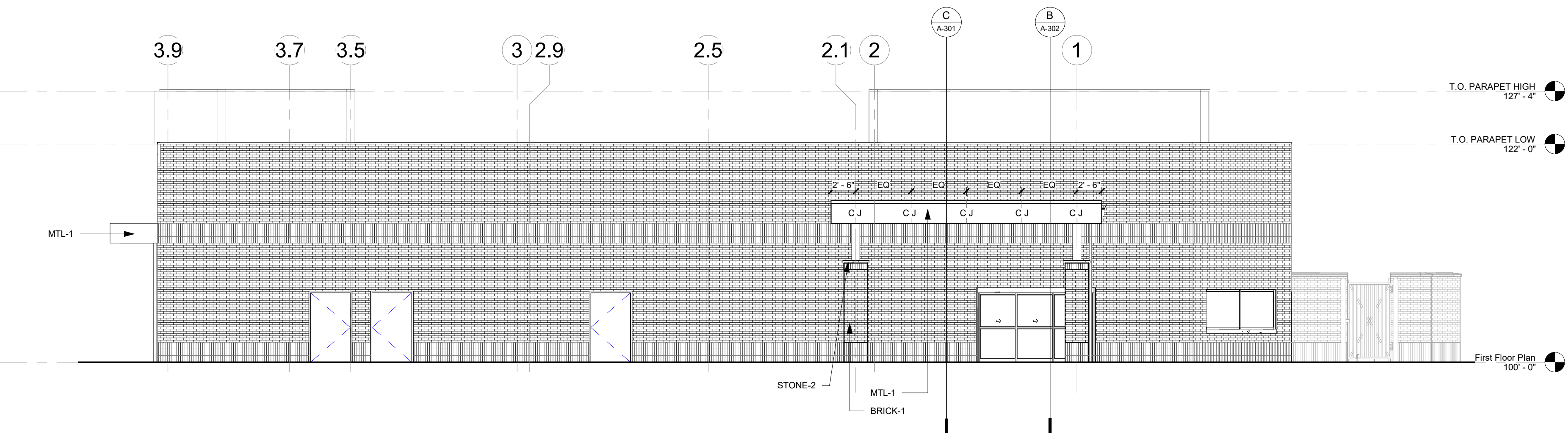
E East Elevation Scale: 1/8" = 1'-0"
