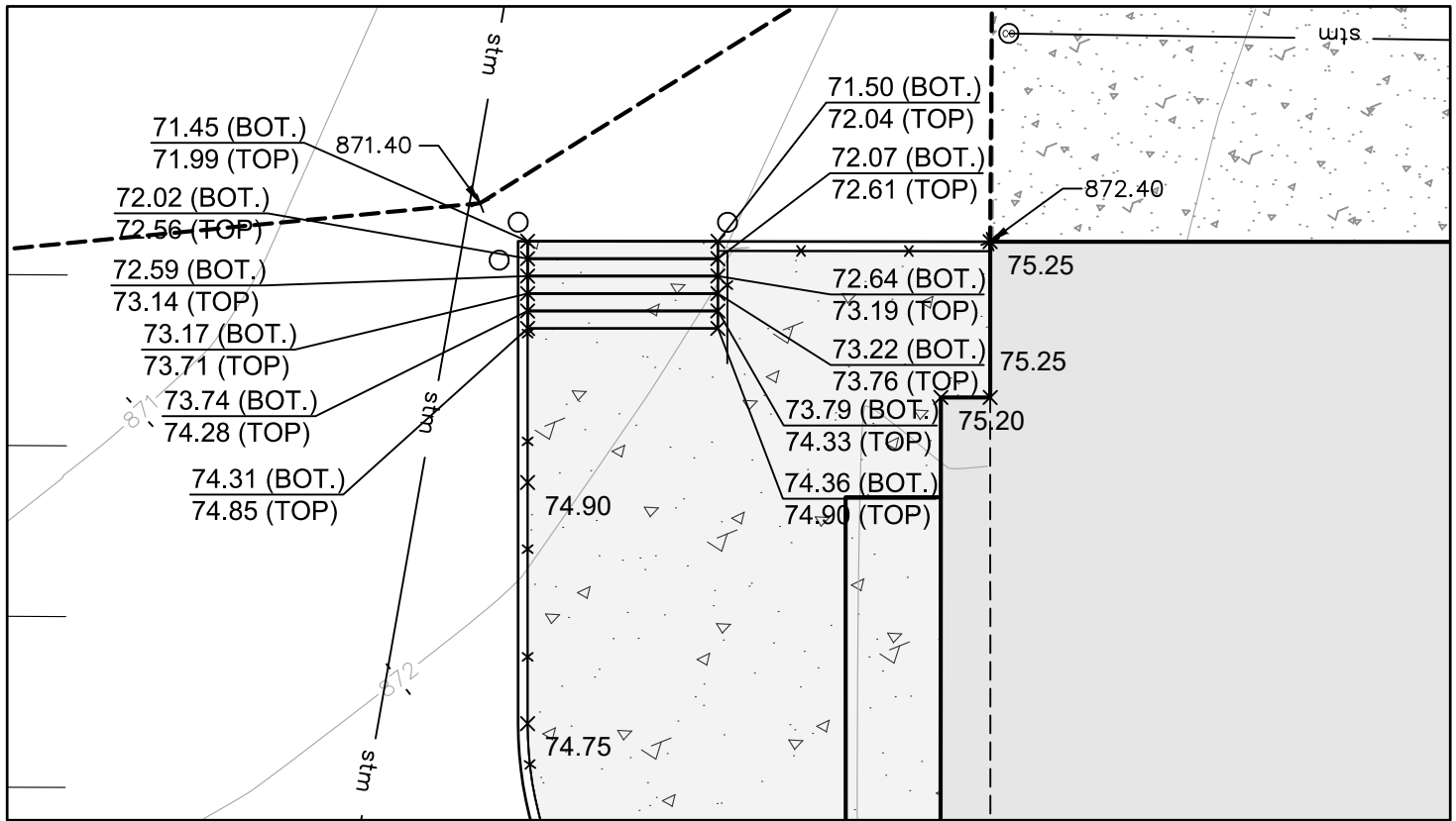
BOT. - BOTTOM OF RISER TOP - TOP OF RISER STAIRWAY DETAIL SCALE: 1" = 10'
