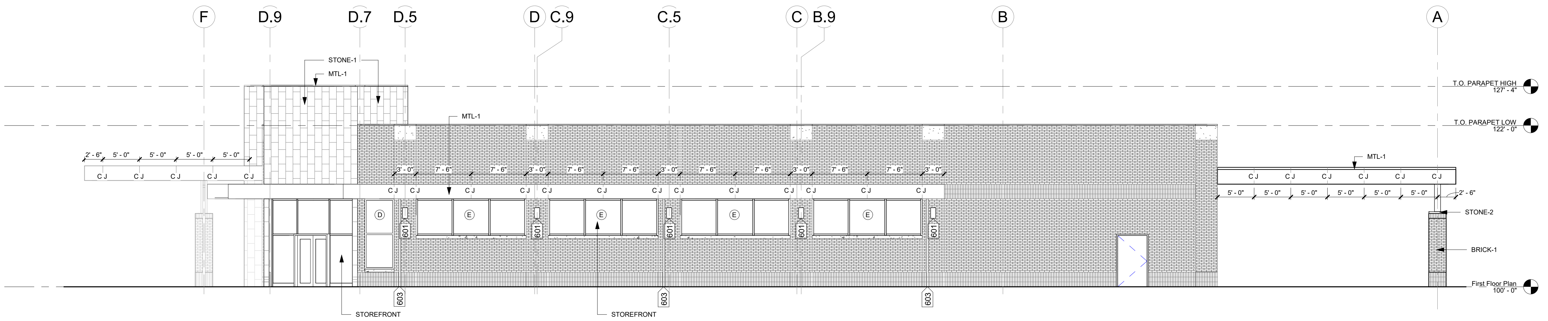
A South Elevation Scale: 1/8" = 1'-0"
